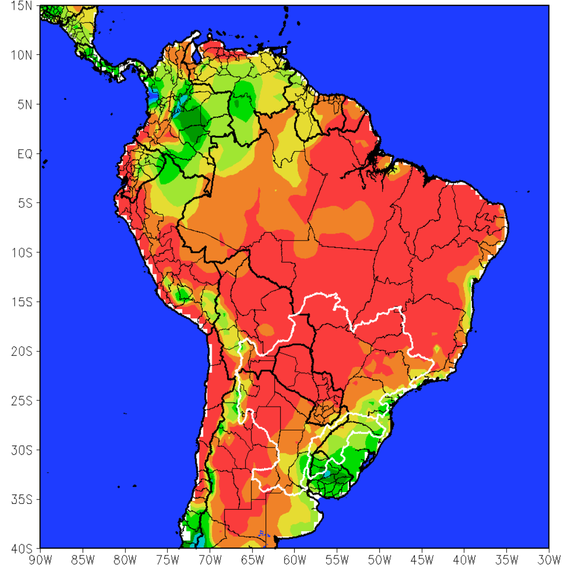
REANALISIS BALANCE HIDRICO ANO 2019 MES 9 CONTENIDO DE AGUA DEL SUELO (%)
