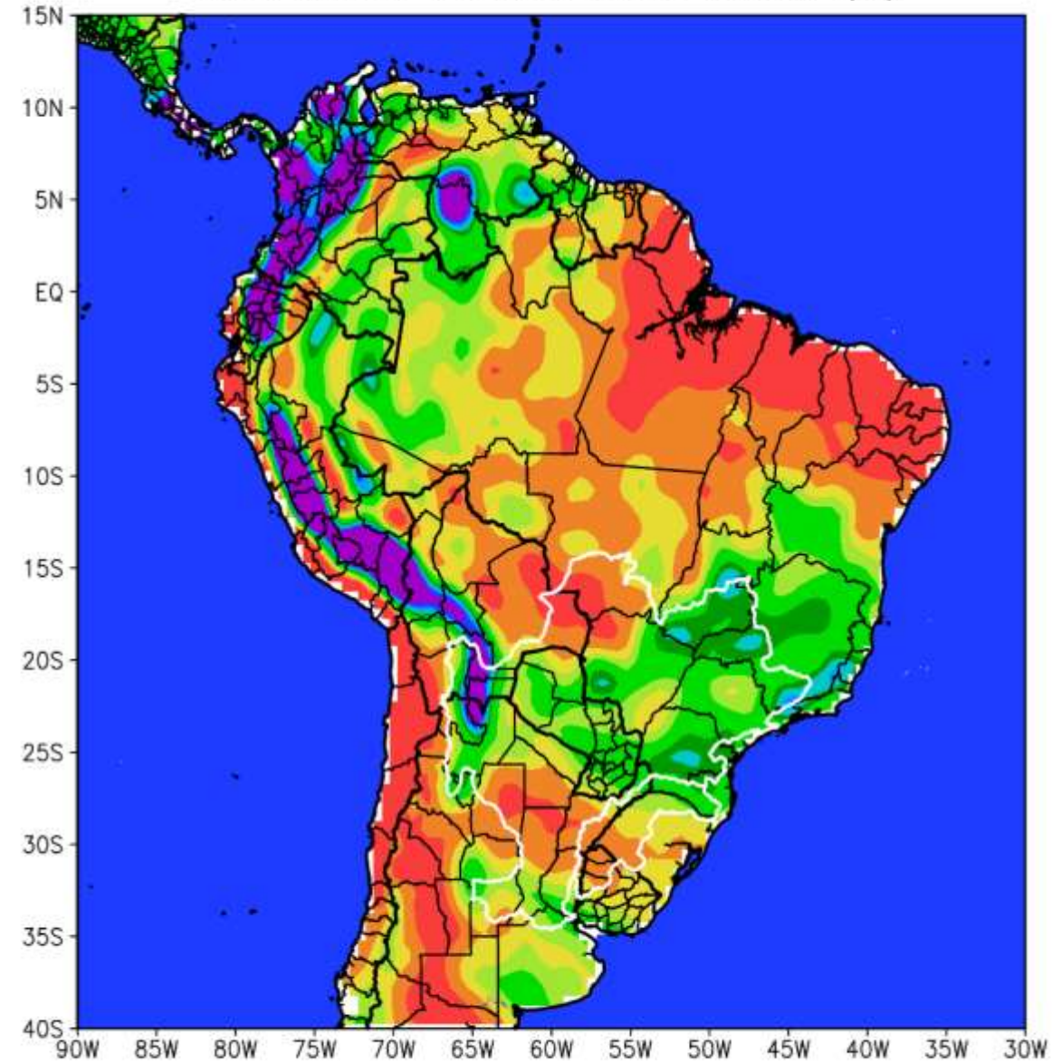
PRONOSTICO BALANCE HIDRICO ANO 2020 MES 11 CONTENIDO DE AGUA DEL SUELO (%)
