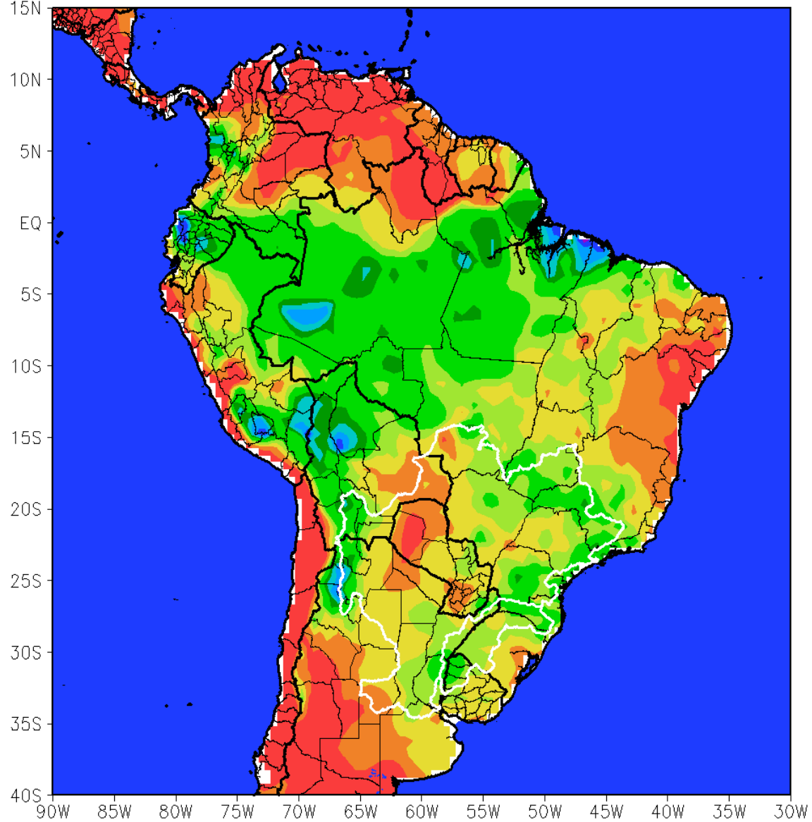
REANALISIS BALANCE HIDRICO ANO 2019 MES 2 CONTENIDO DE AGUA DEL SUELO (%)
