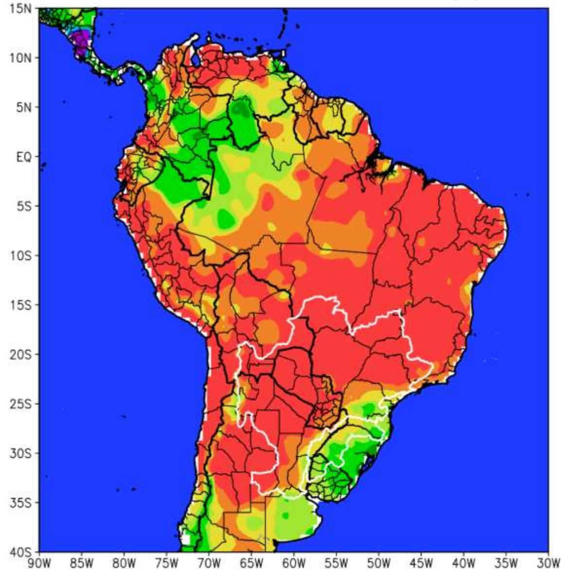
REANALISIS BALANCE HIDRICO ANO 2020 MES 10 CONTENIDO DE AGUA DEL SUELO (%)
