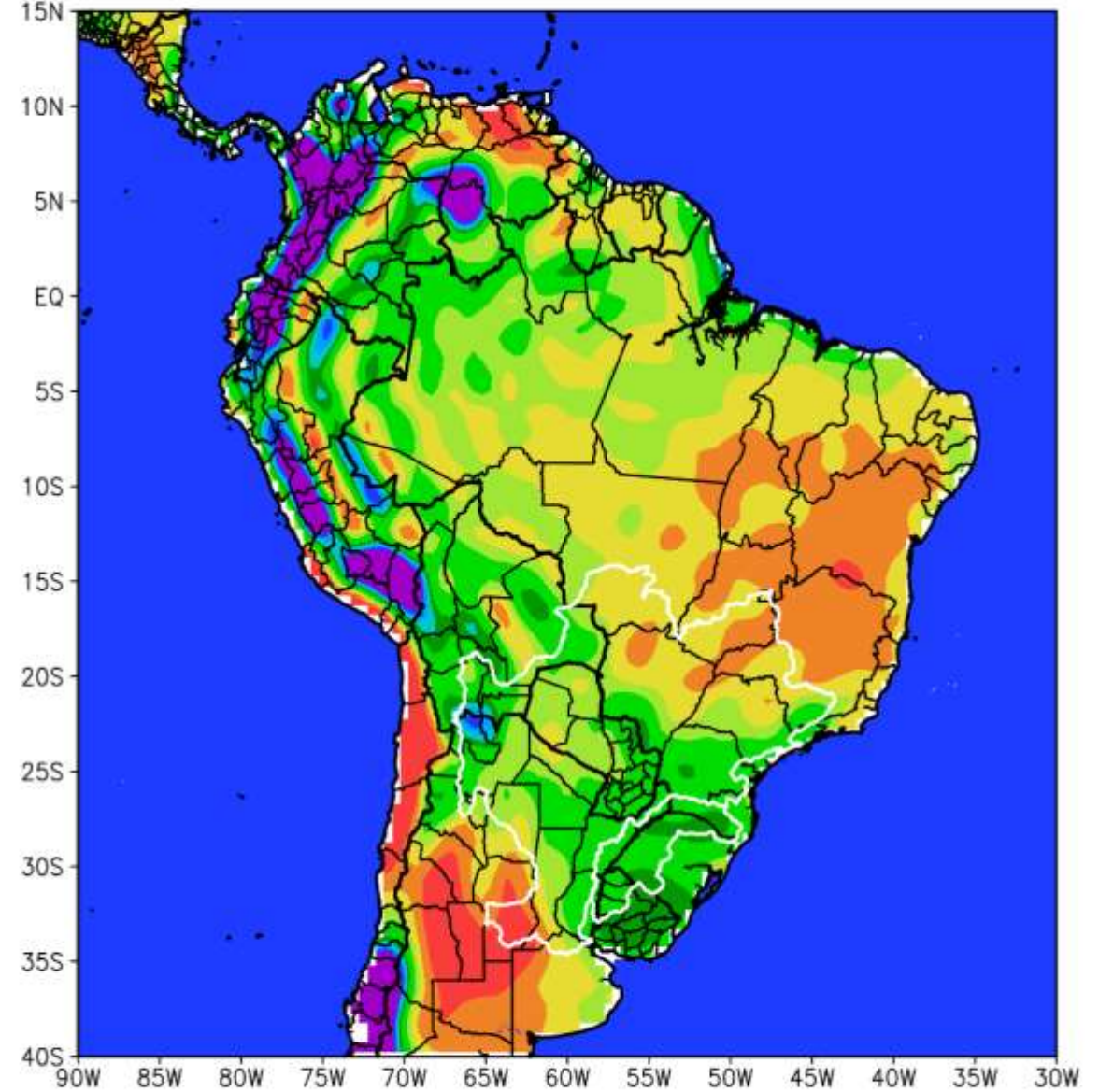
PRONOSTICO BALANCE HIDRICO ANO 2021 MES 5 CONTENIDO DE AGUA DEL SUELO (%)
