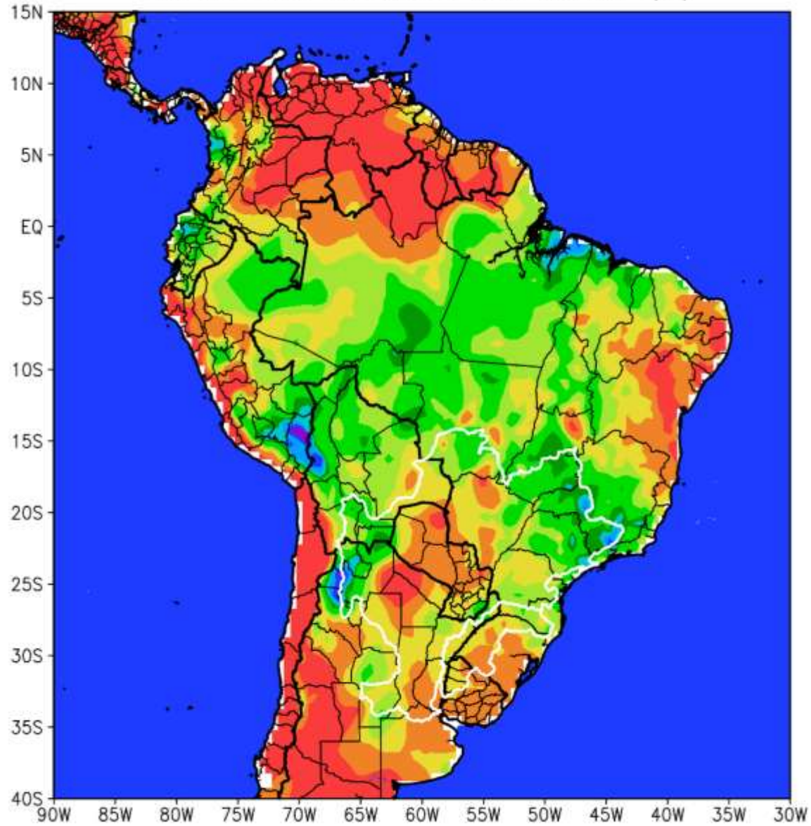
REANALISIS BALANCE HIDRICO ANO 2020 MES 2 CONTENIDO DE AGUA DEL SUELO (%)
