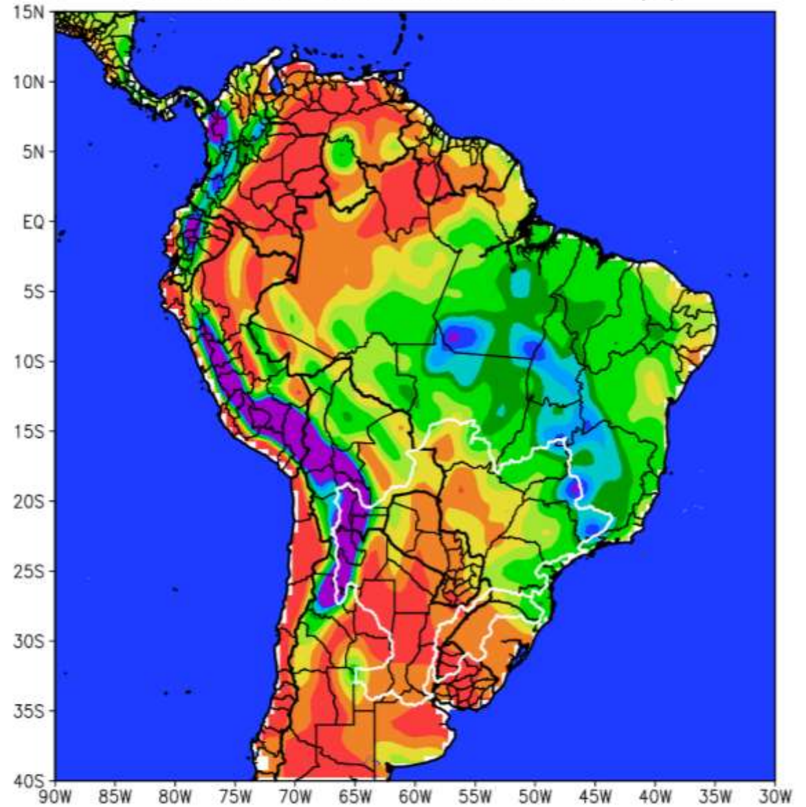
PRONOSTICO BALANCE HIDRICO ANO 2021 MES 1 CONTENIDO DE AGUA DEL SUELO (%)
