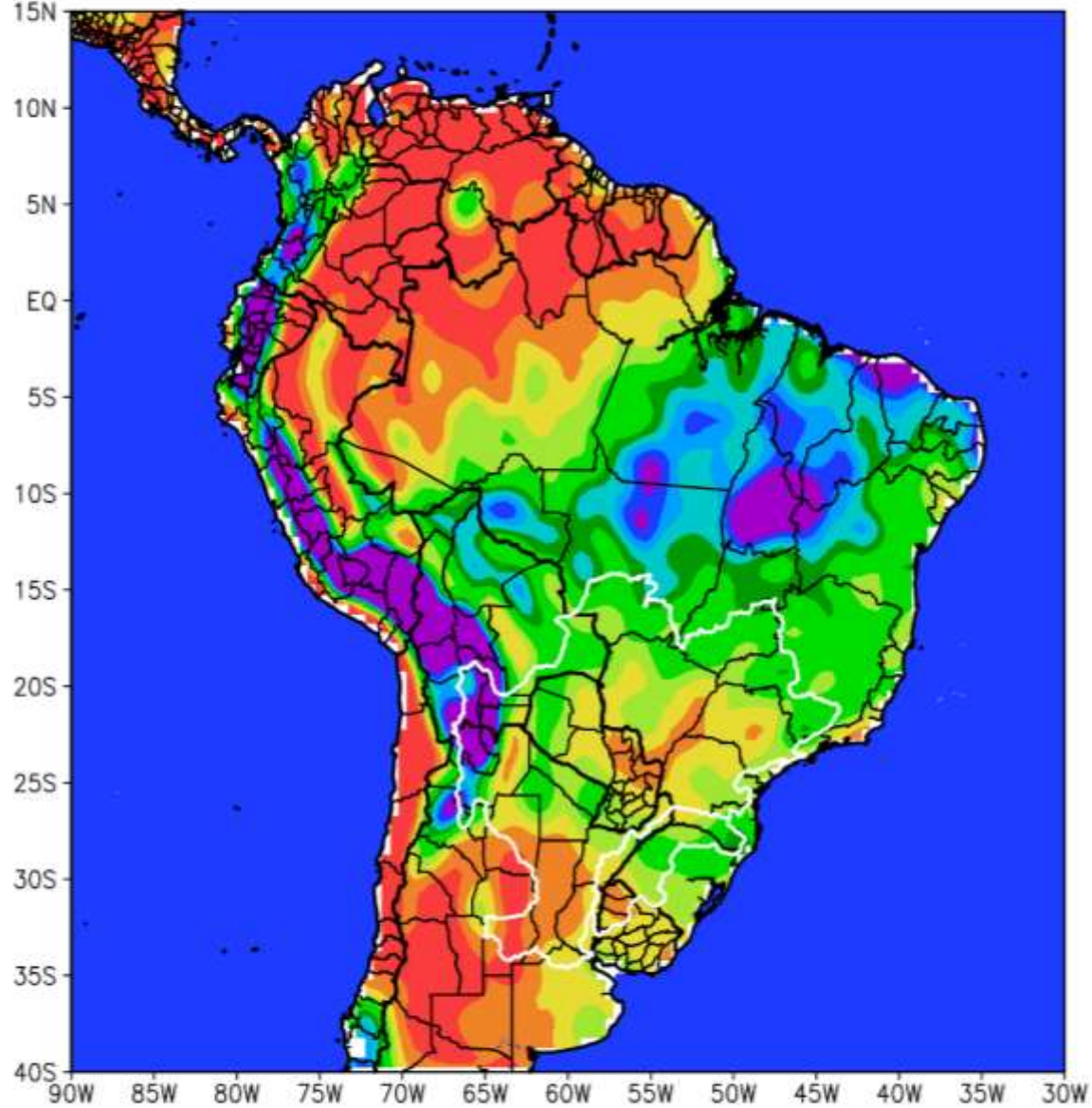
PRONOSTICO BALANCE HIDRICO ANO 2021 MES 3 CONTENIDO DE AGUA DEL SUELO (%)
